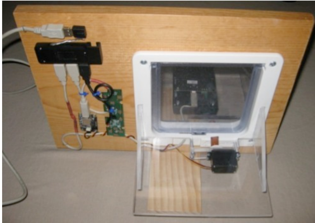
Twitter Enabled Cat Door
